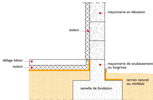
CONSTRUCTION AVEC RUPTEUR THERMIQUE - élévation maçonnerie ( agglo) - SUR TERRE PLEIN
