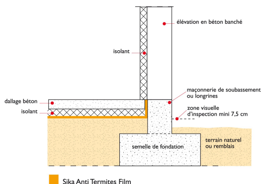
DALLE DÉSolidARISÉE SUR TERRE PLEIN AVEC ISOLANT SOUS DALLAGE
