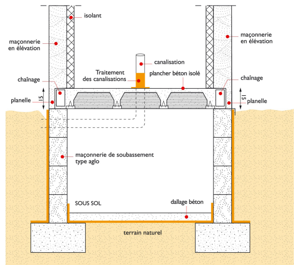
CONSTRUCTION SUR SOUS-SOL
