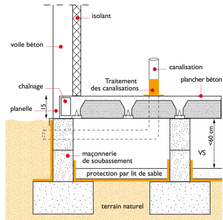
CONSTRUCTION SUR VIDE SANITAIRE < 60 cm
