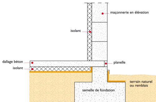
DALLE PORTÉE SUR TERRE PLEIN AVEC ISOLANT SOUS DALLAGE
