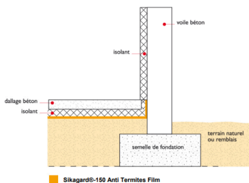
ELEVATION BÉTON ARMÉ (bouché)
