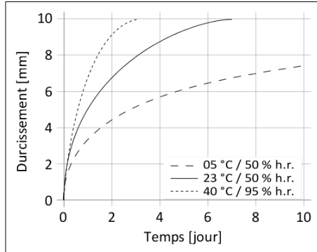
Schéma 1: Vitesse de polymérisation du Sikasil® WS-605 S
